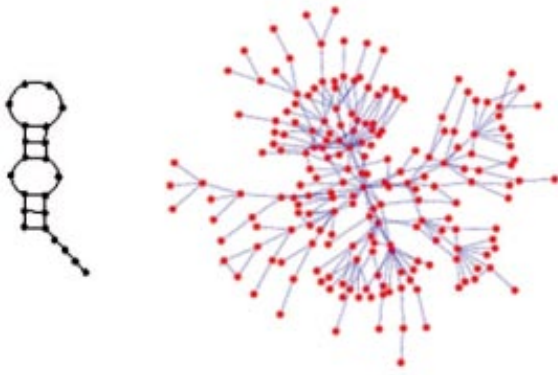
Figura 2. Una estructura simple de RNA (izquierda) a la que acompaña una representación esquemática de la red neutral correspondiente (derecha). Los nodos en rojo representan secuencias cuya estructura plegada de mínima energía es la mostrada. Las aristas unen cada par de nodos que difieren en una única mutación, es decir, dos moléculas que se diferencian en un solo nucleótido.
